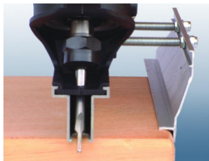
Nutfräsung 90° und Parallelanschlag
